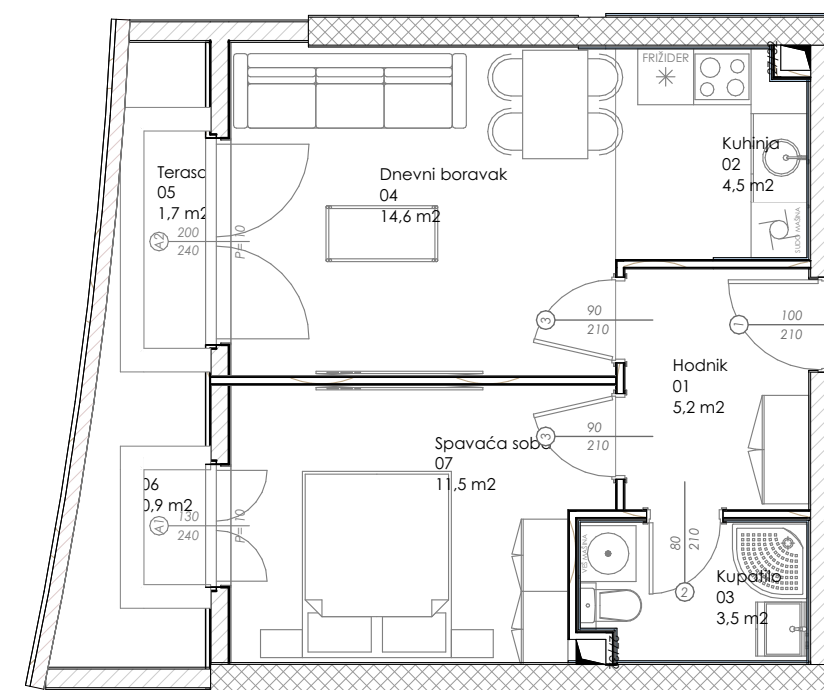
ORGANIZACIJA STANA L1-I-J2
